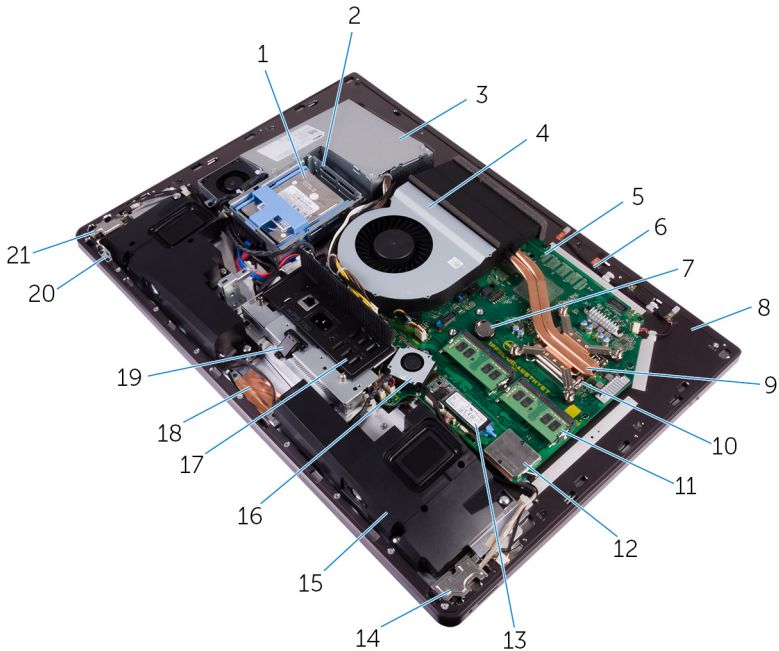
Kuva 1. : Tietokone sisältä
